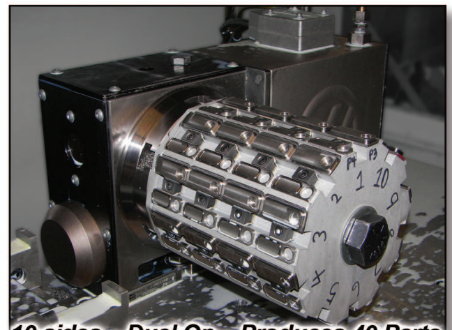
10 sides – Duel Op – Produces 40 Parts
